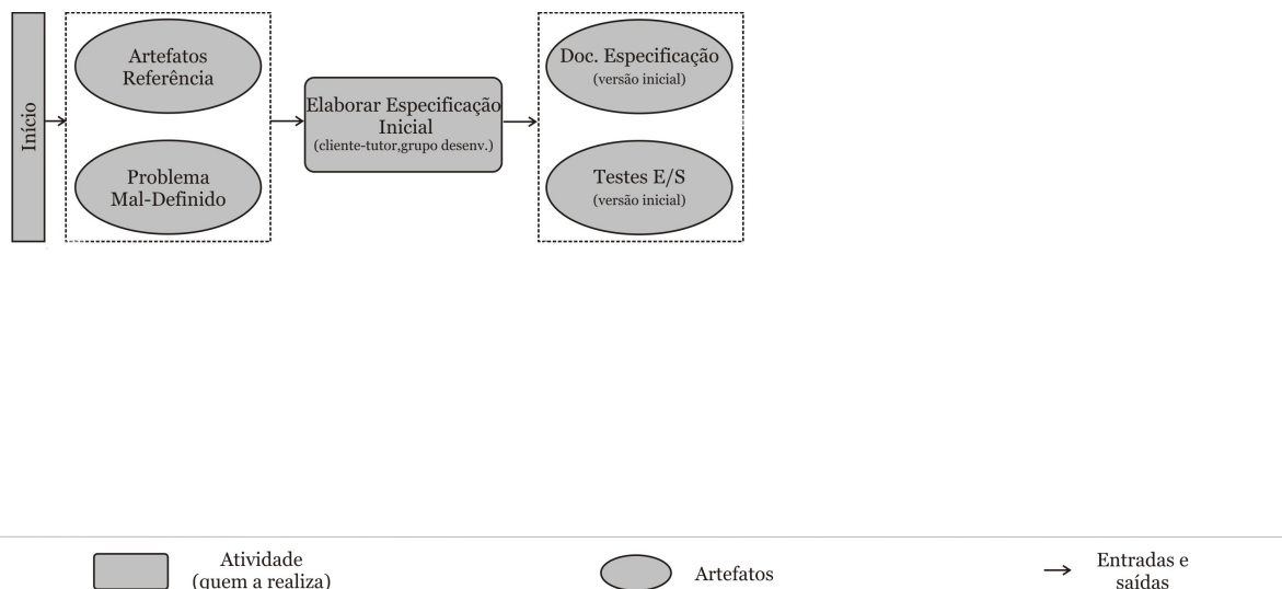
Figura 3.2: Atividade: Elaborar especificação inicial.
