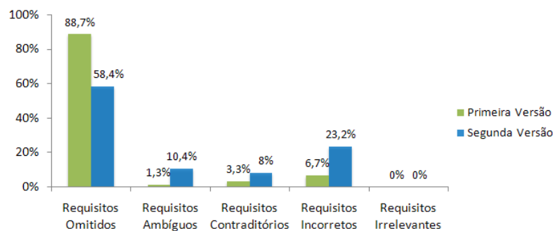
Figura 5.13: Grupo POP – Tipos de defeitos encontrados na primeira versão do documento.
