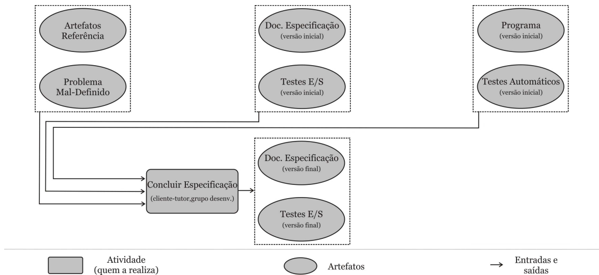
Figura 3.4: Atividade: Concluir especificação.
