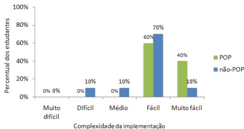
Figura 5.9: Complexidade da implementação segundo os estudantes.
