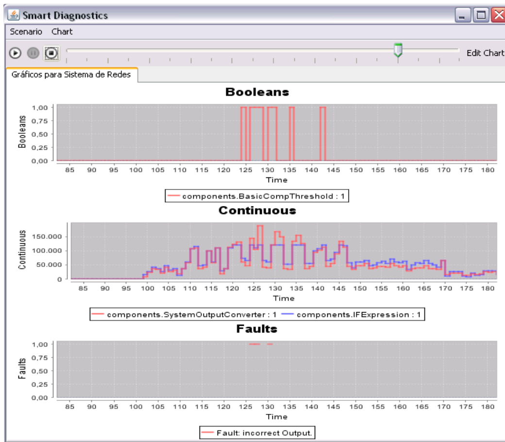
Figura 35: Falha no Modelo do bloco REENGINE com Limite de Banda.
