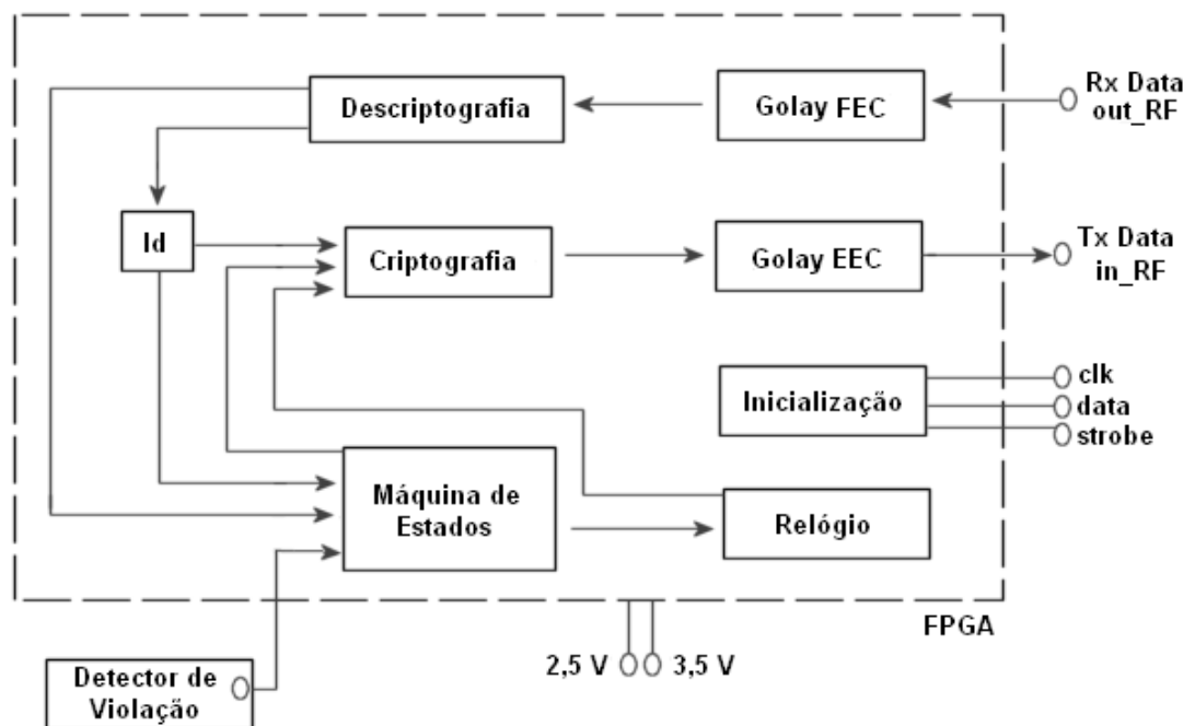
Figura 24: Diagrama de Blocos do Lacre Digital.
