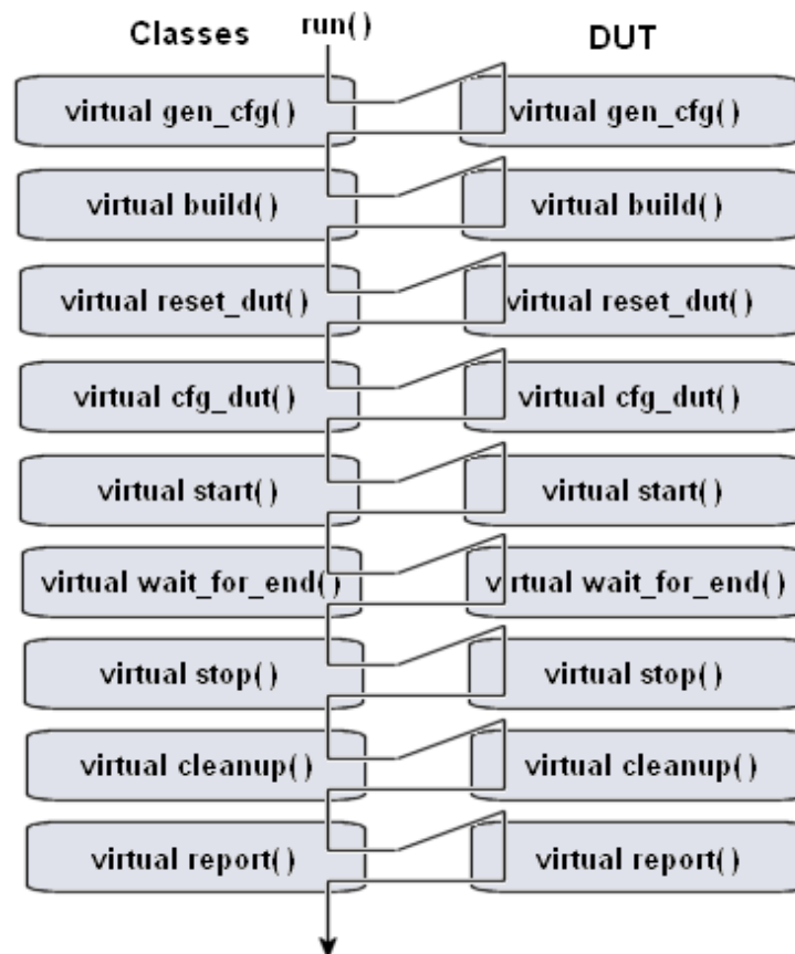
Figura 03: Definição da classe vmm_env com métodos virtuais.
