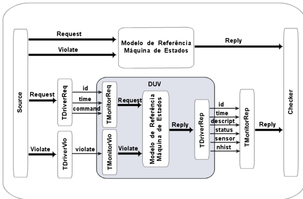
Figura 13: Testbench do bloco Máquina de Estados.
