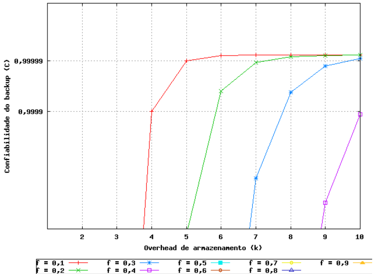
Figura 2 – Cinco noves de confiabilidade ( C = 0,99999 )
