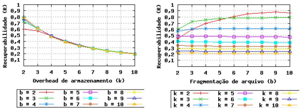
(a) S = 10\text{GB} , d = 300\text{Kbps} e u = 150\text{Kbps} para diferentes valores de b
