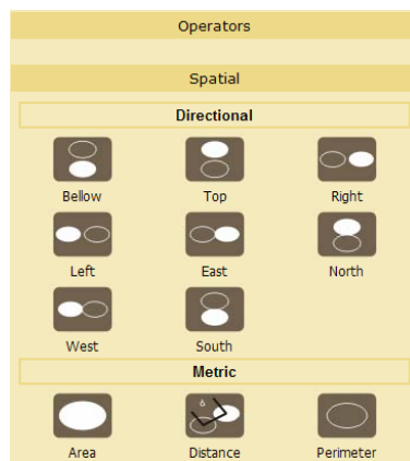
Figura 65: Operadores Espaciais .
