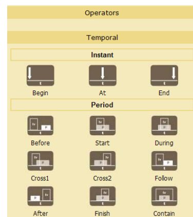
Figura 66: Operadores Temporais.
