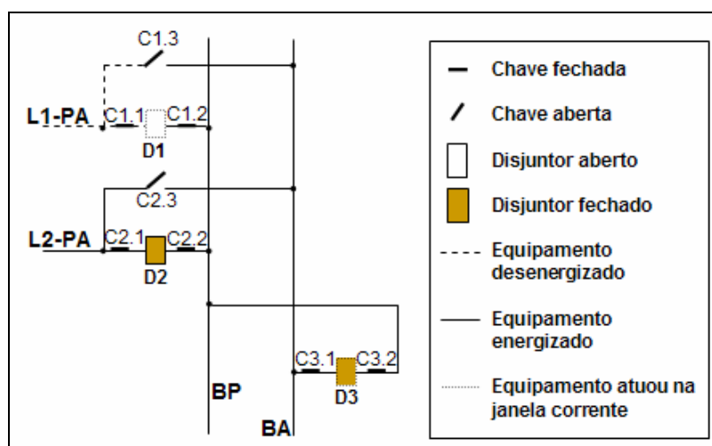
Figura 4.14 – Estado do modelo diante de eventos com ruído relacionados com uma manobra de bypass
