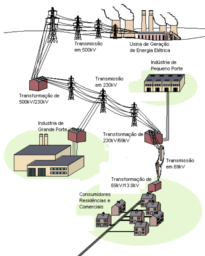
Figura I-3: Esquema típico de transmissão e distribuição de energia
