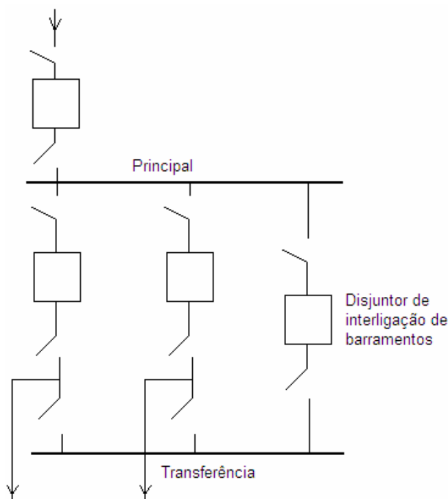
Figura I-11: Arranjo com barramento principal e de transferência
