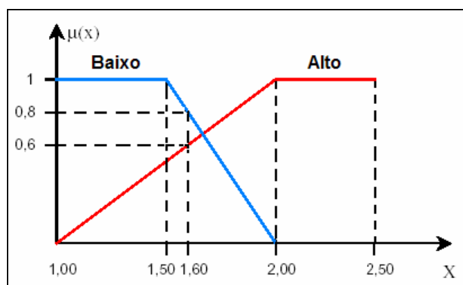
Figura 3.2 – Conjuntos nebulosos
