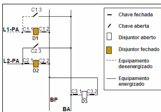
Figura 2.8 – Estado dos equipamentos após o desligamento da linha L1 (evento de abertura do disjuntor D1 foi perdido)
