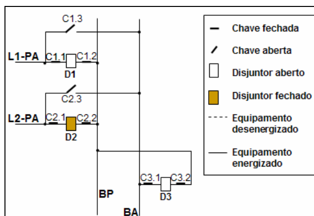
Figura 2.9 – Estado dos equipamentos após o religamento (evento de fechamento do disjuntor D1 foi perdido)
