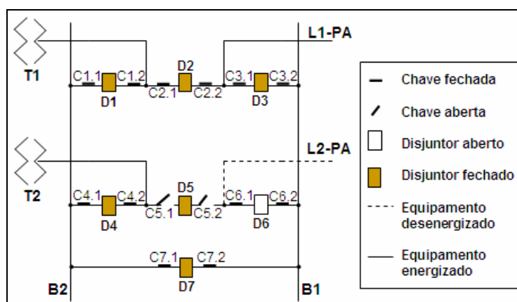
Figura 2.2 – Exemplo de um arranjo
