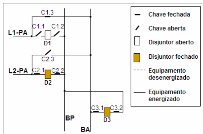
Figura 2.10 – Estado dos equipamento após a realização do bypass
