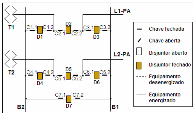
Figura 2.3 - Estado dos equipamentos antes do desarme
