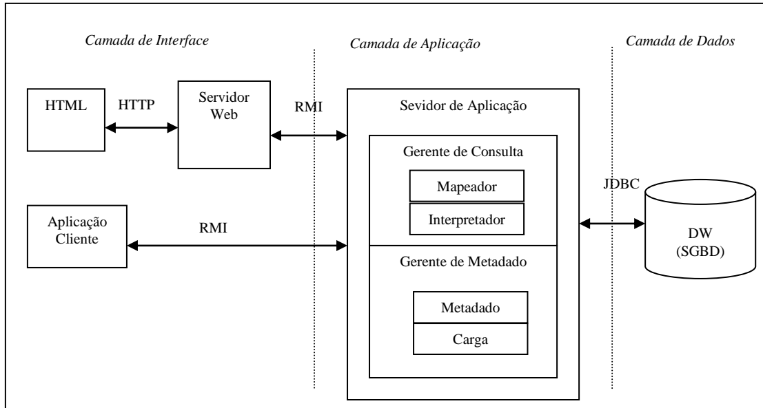
Figura 5.1: Projeto Arquitetural do S-DW-E.
