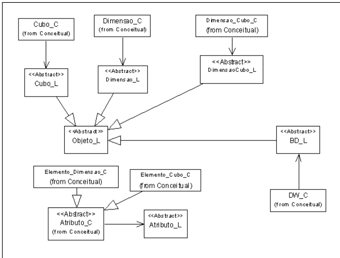
Figura 5.4: Diagrama de classes UML do modelo de metadados lógico do framework.
