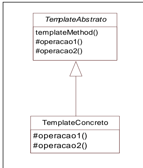
Figura 3.5: Padrão Template Method
