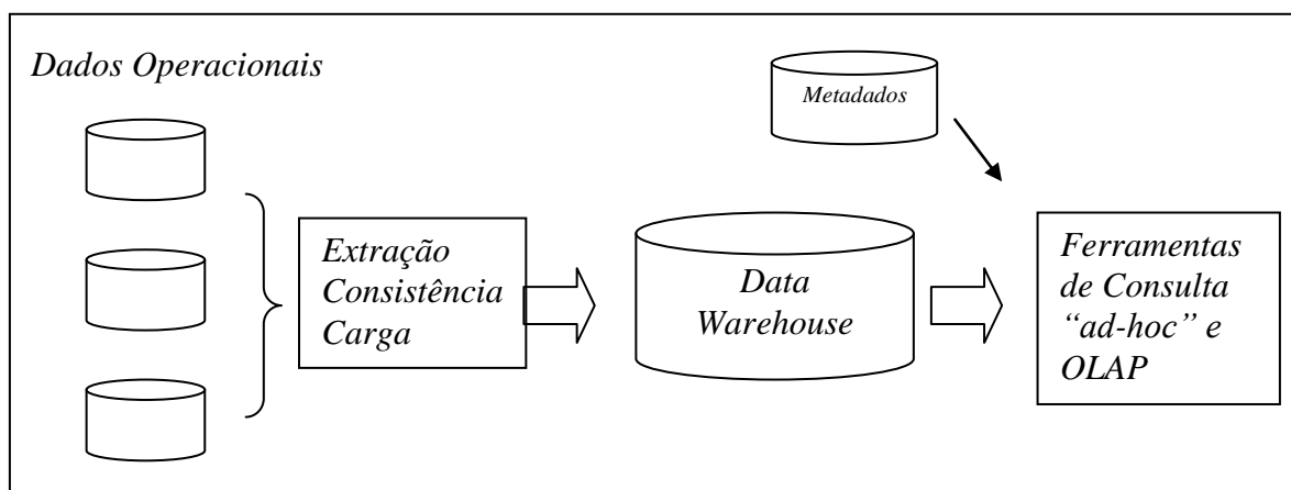
Figura 2.1: Arquitetura genérica de um sistema de DWing
