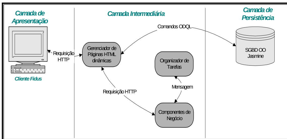
Figura 4.2: Camadas da arquitetura do Fidus.
