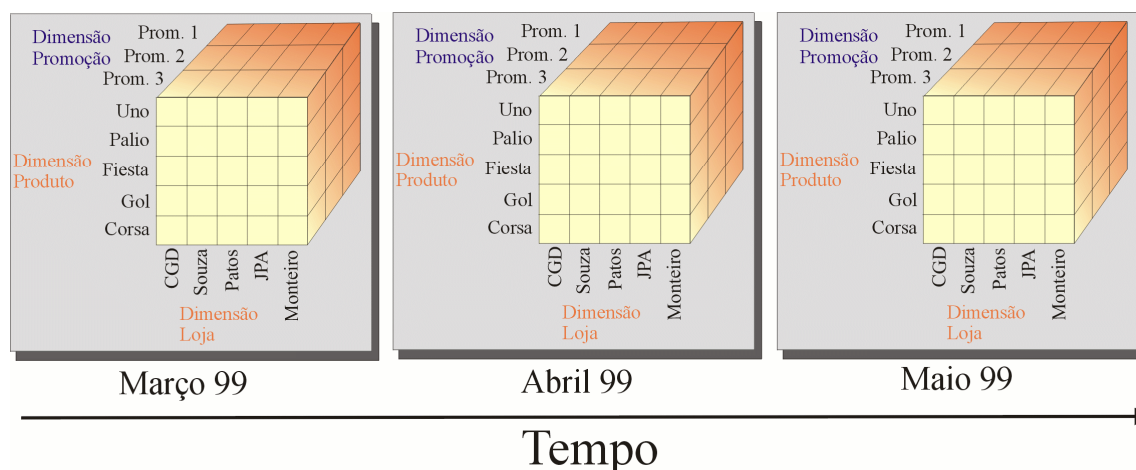
Figura 2.3 - Cubo quadridimensional.
