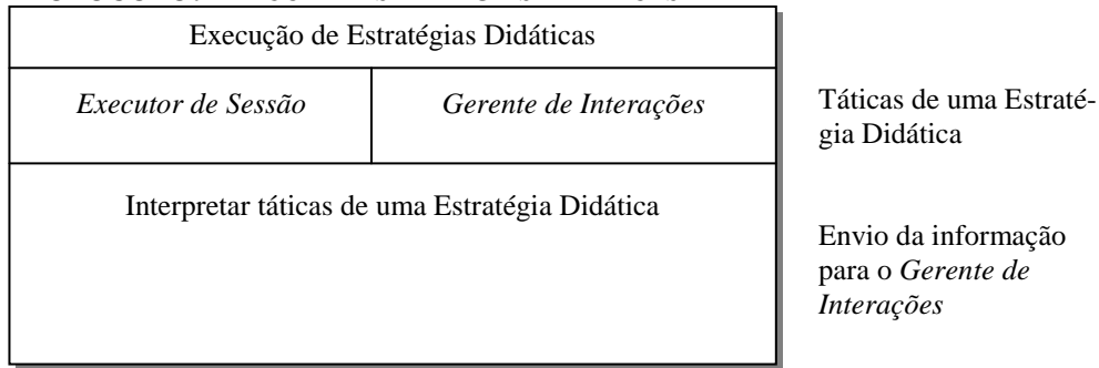
Figura 5.11: Definição do Protocolo ExecutarEstratégiasDidáticas
