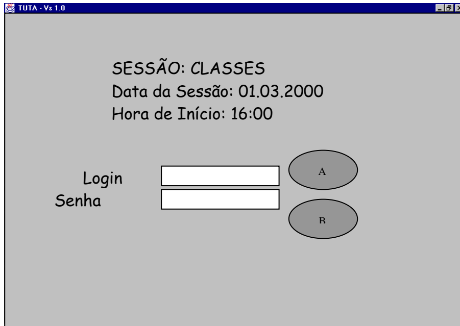
Figura 5.15: Interface referente ao caso de uso IniciarSessão
