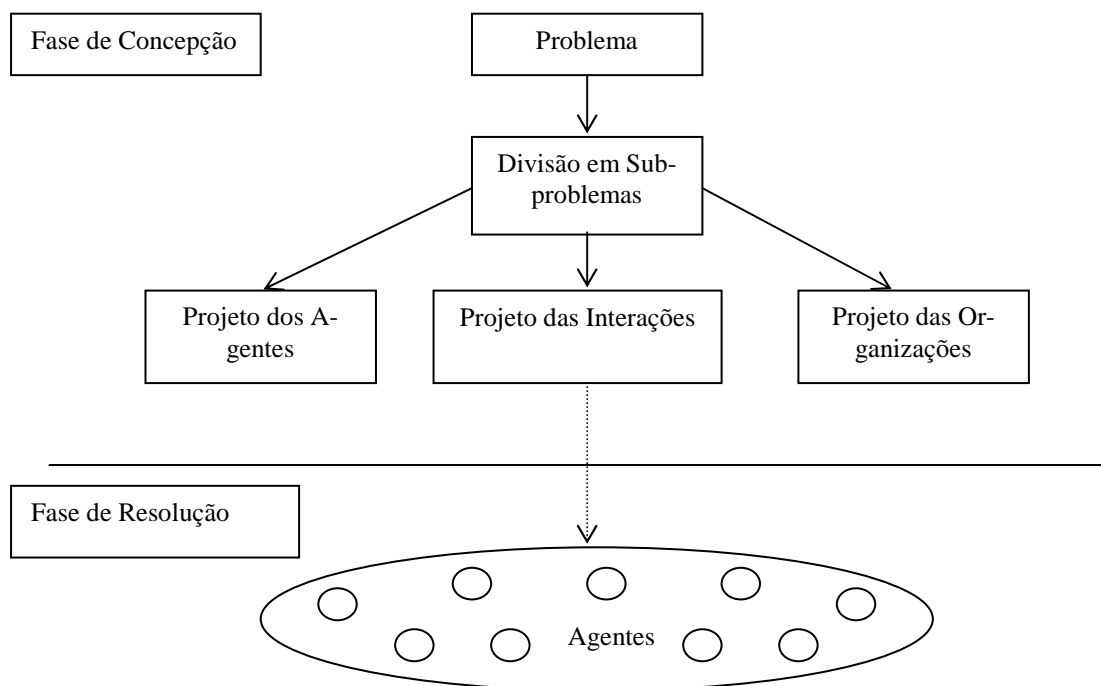
Figura 3.2: Abordagem RDP
