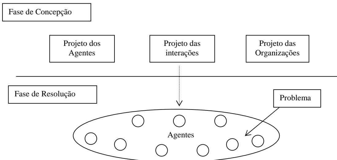
Figura 3.3: Abordagem SMA
